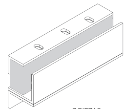
PERFIL 'ZL' 'ZL' PROFILE
