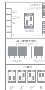
CABLEADO WIRING
